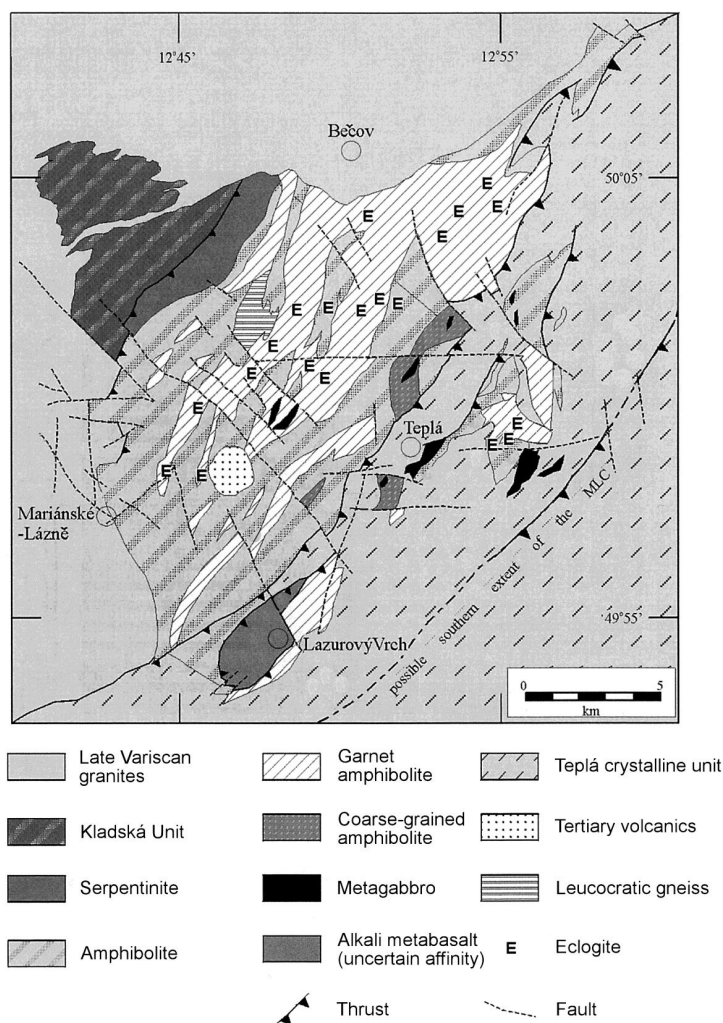
■ Fig. 3. Geological map of the Mariánské Lázně Complex (modified from Crowley et al., 2002, after Jelínek et al., 1997).
